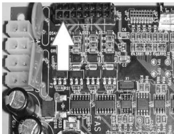
Détail connecteur JP2
