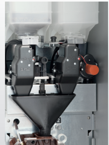
Regulación automática del molido en caffè Top (en la versión con doble campana)
